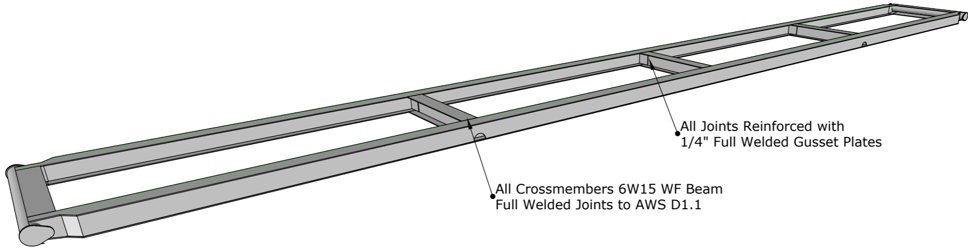
2 4ftx40ft Rig Mat
