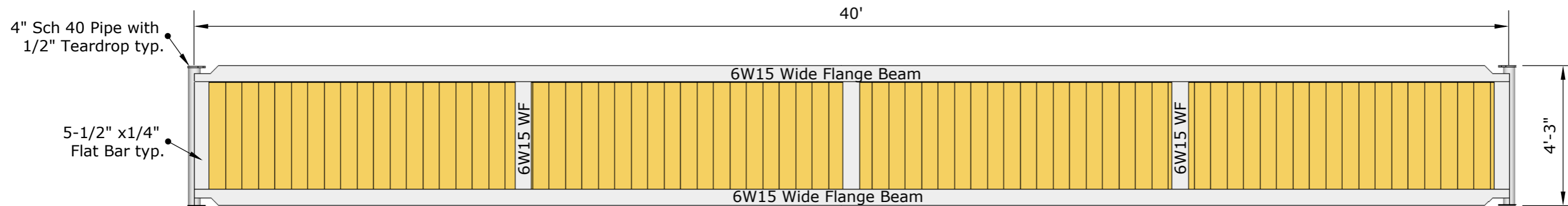
2 4ftx40ft Rig Mat Dimensions Scale: 1:40
