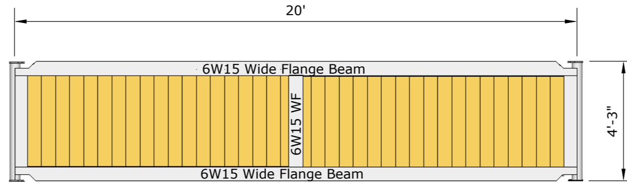
1 4ftx20ft Rig Mat Dimensions Scale: 1:40
