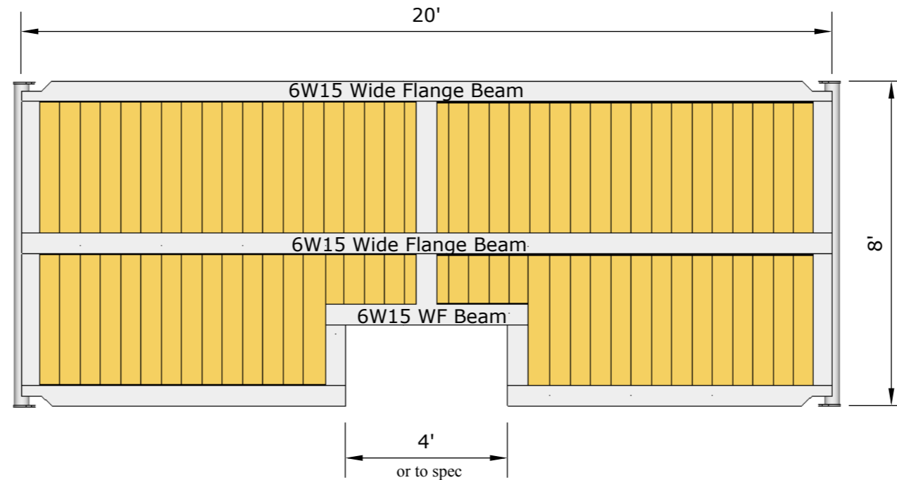
1 8ftx20ft Rig Mat Dimensions Scale: 1:40
